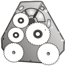
Gehäuseblock G komplett Housing unit G cpl.
